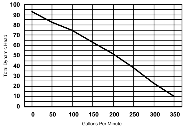
Piranha Model PS-1000-A 10 HP 230/460 Volt
